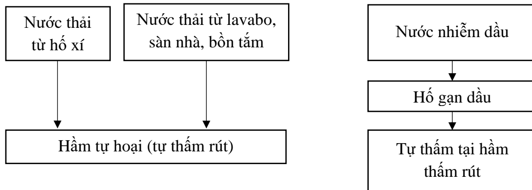
Hình 3. Sơ đồ thu gom và thoát nước thải tại cơ sở
